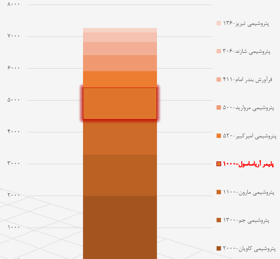
ظرفیت تولید اتیلن در ایران (هزار تن در سال)
