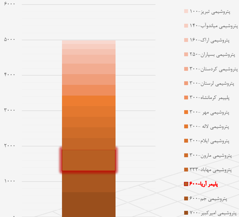
ظرفیت تولید پلی اتیلن در ایران (هزار تن در سال)
