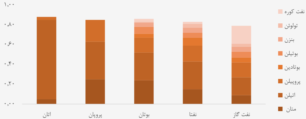
درصد تبدیل محصولات بر اساس خوراک ورودی
